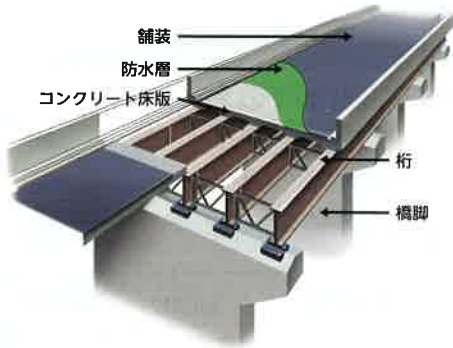
鋼橋の構造
